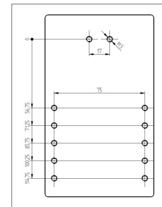
Bild 3: Bohrbild
