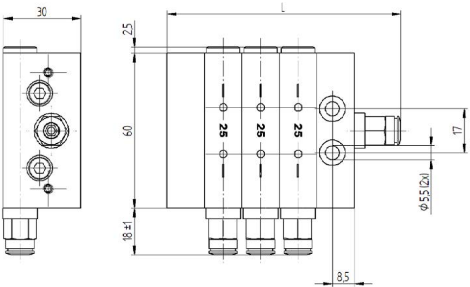
Abb. 1: Prinzipskizze PRV-3
