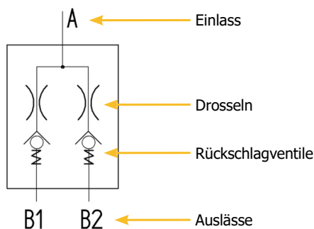
Hydraulisches Schaltbild des Splitter 1:2
